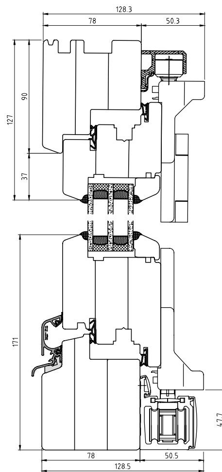
BI-FOLDING DOOR WOOD CLASSIC VI 78
